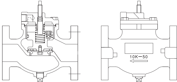
図1:YVB型（バタフライ弁無し）
