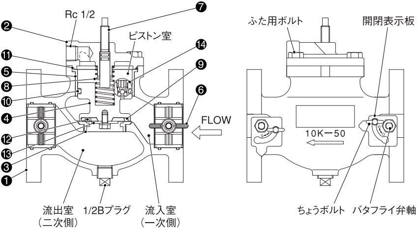
バタフライ弁 作動図
