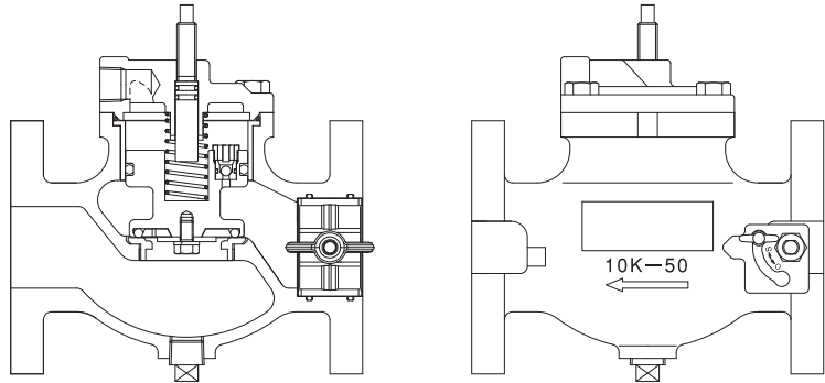
図2:YVB-V型（片側バタフライ弁）
