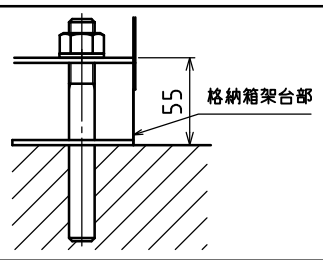
アンカーボルト取付状態例
