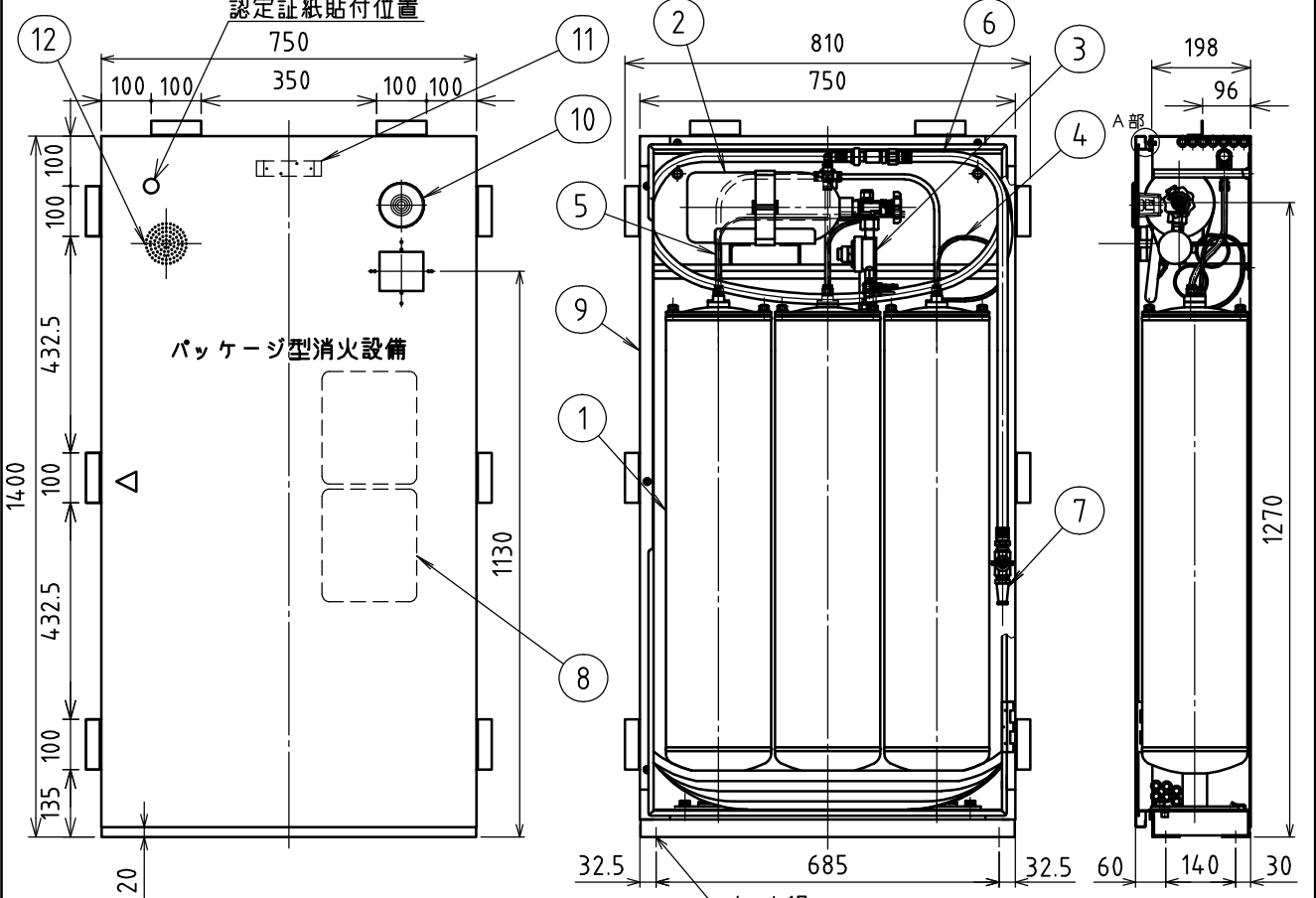
アンカーボルト取付状態例
