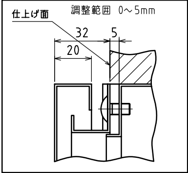
アンカーボルト取付状態例
