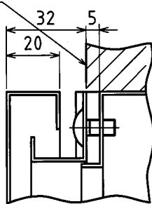
A部詳細図
