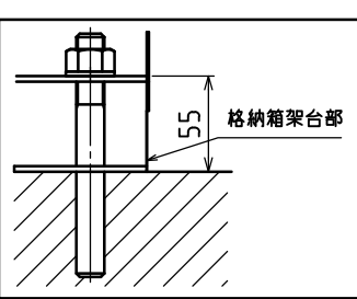
アンカーボルト取付状態例
