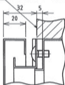
A部詳細図
