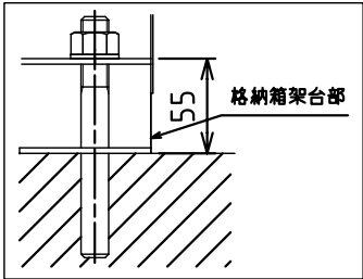
アンカーボルト取付状態例
