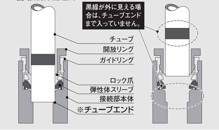
※A図:接続部構造図
