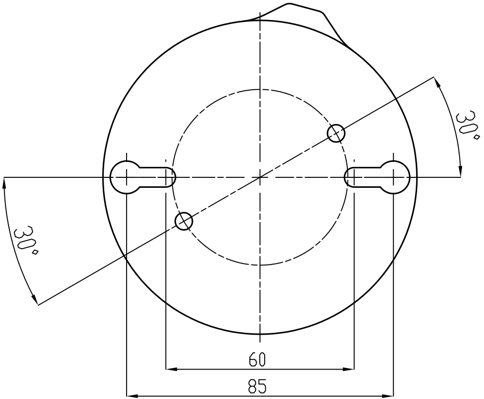
取付穴図（天井側）
