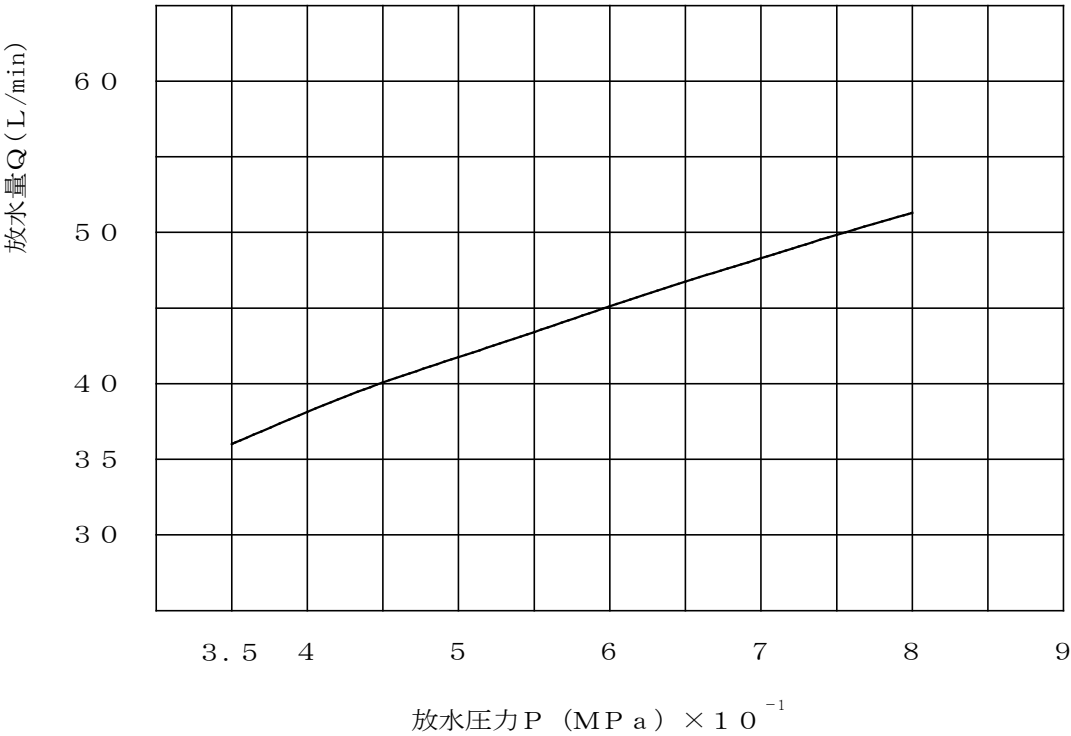
放水量特性P-Q曲線
