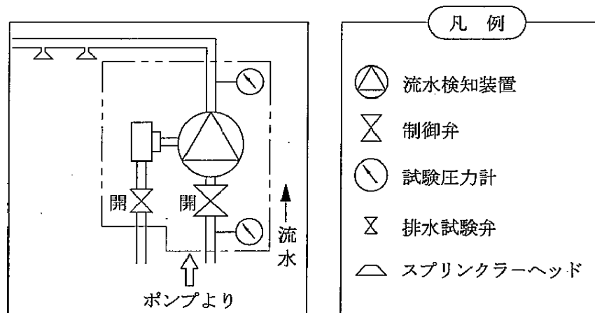
図 10 末端試験
