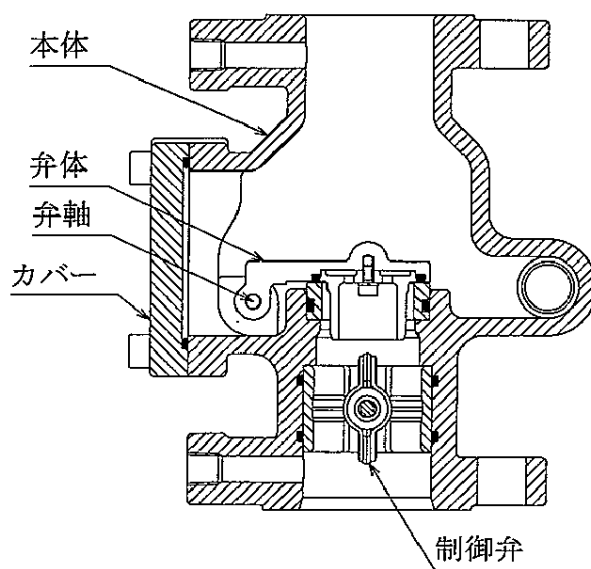
図3 弁本体
