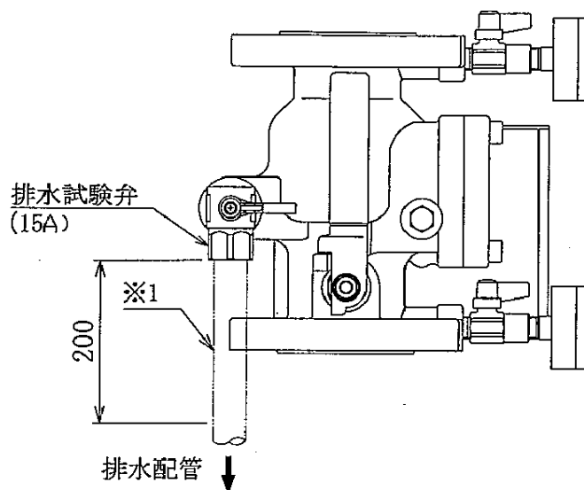
図 15 排水用配管の接続
