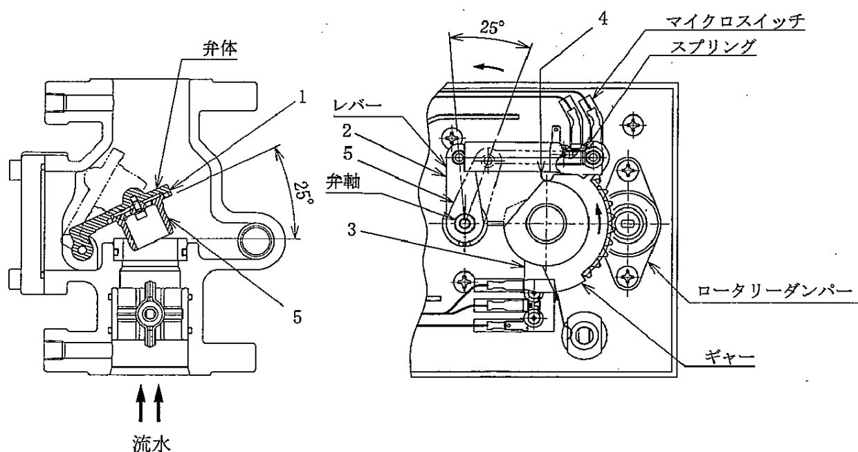
図 7 流水検知装置作動の流れ
