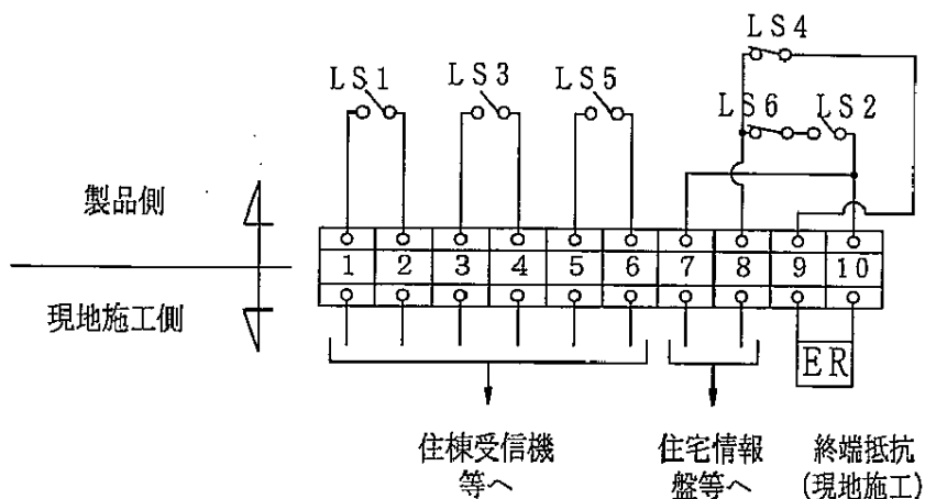
図 14 端子台ユニット結線図
