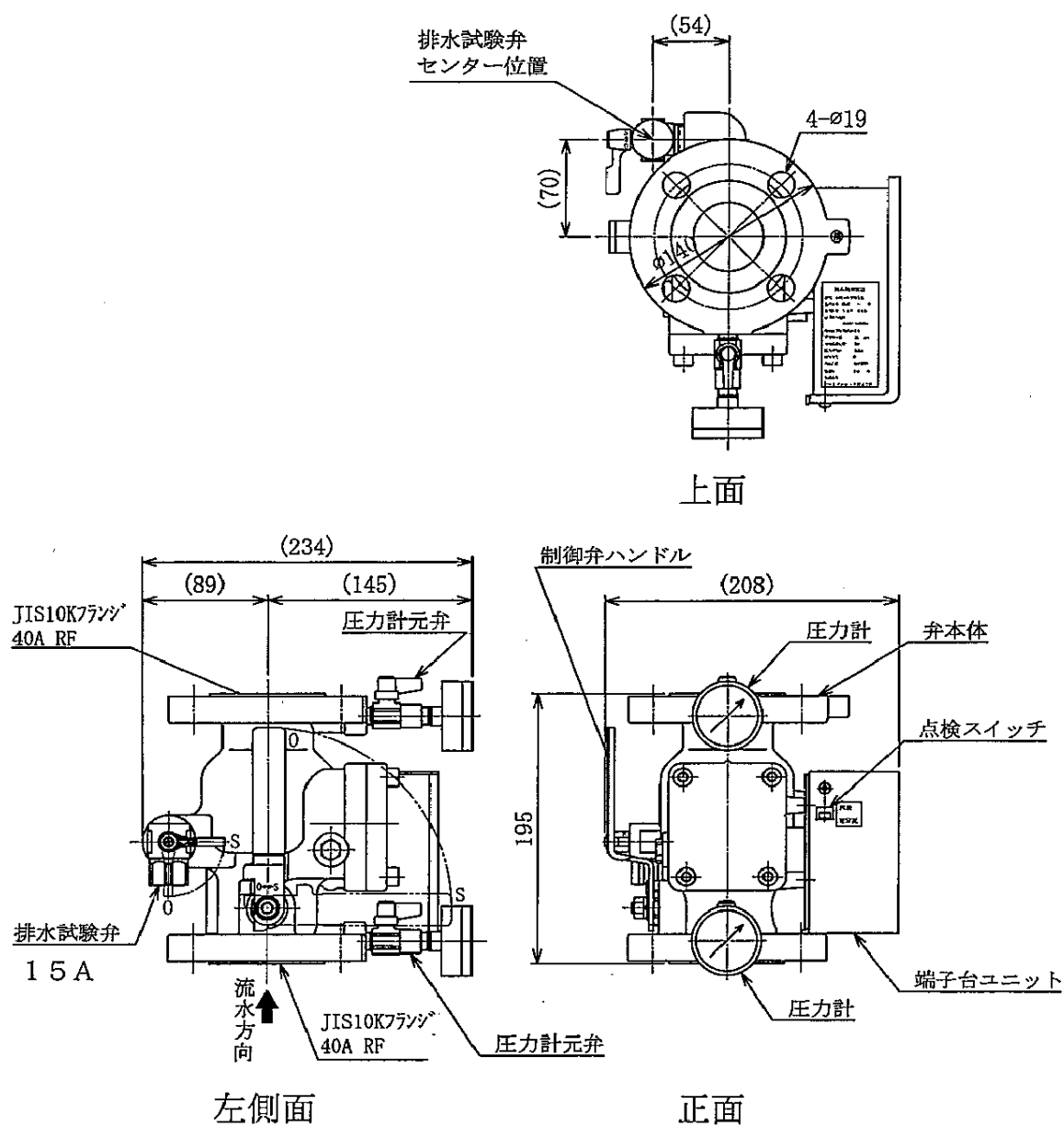
図1 ユニット構成品の名称、外観寸法
