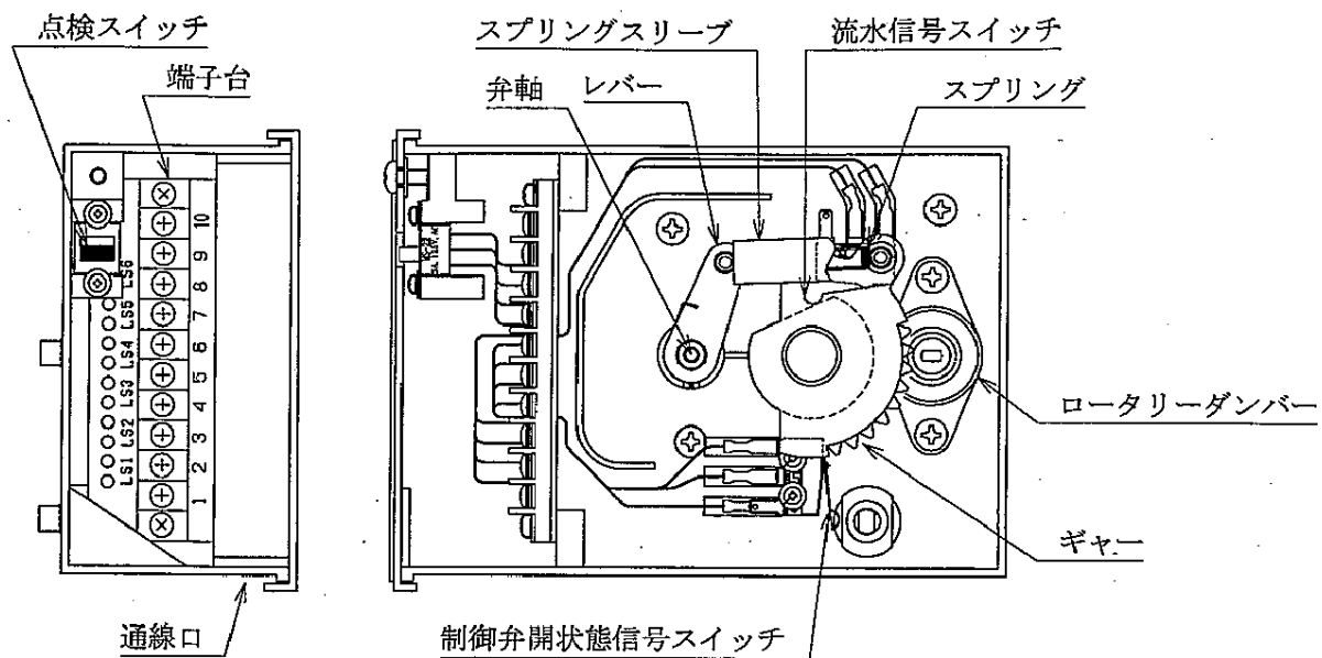
図2 端子台ユニット
