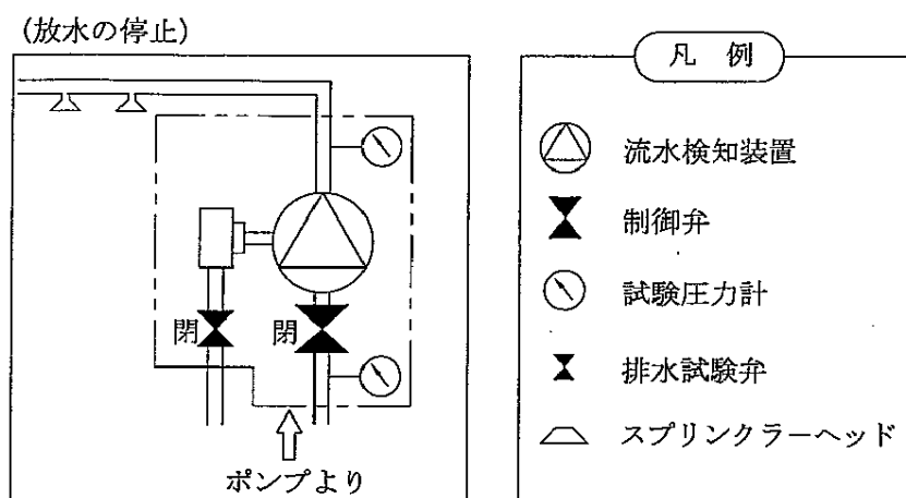
図 8 放水の停止
