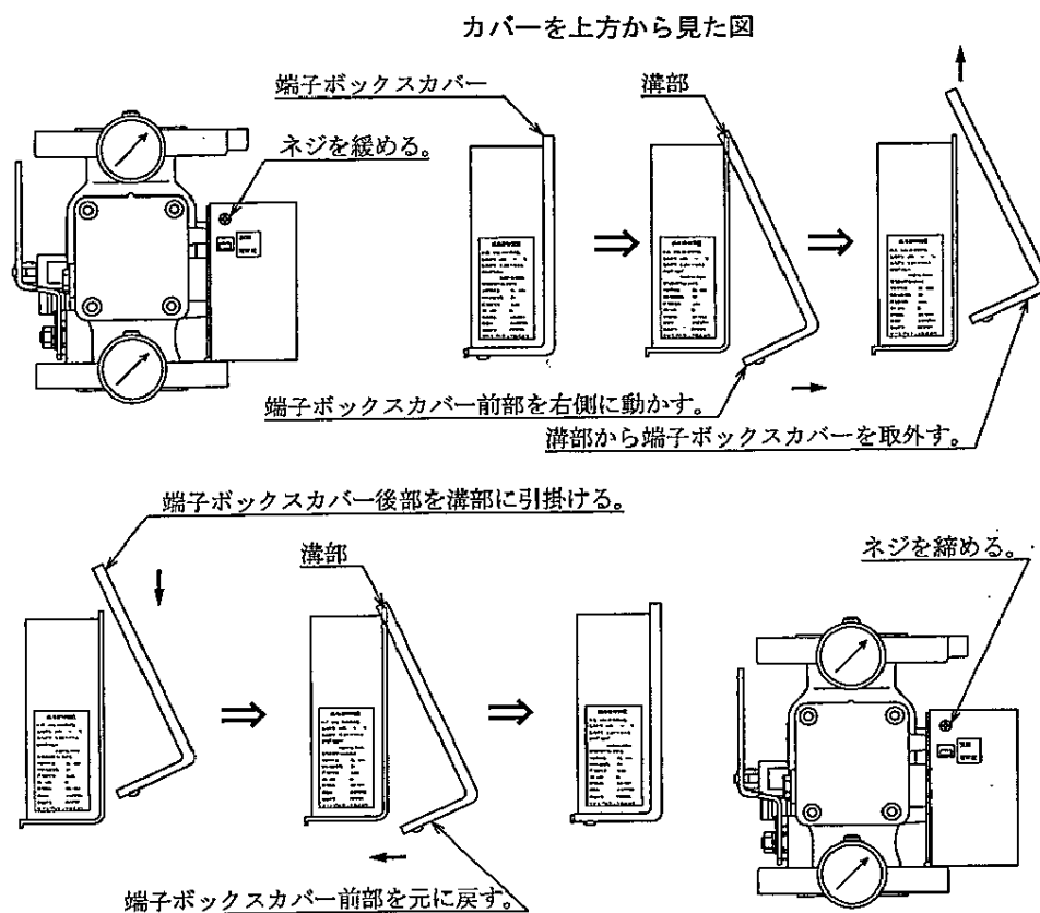
図5 端子ボックスのカバー脱着方法
