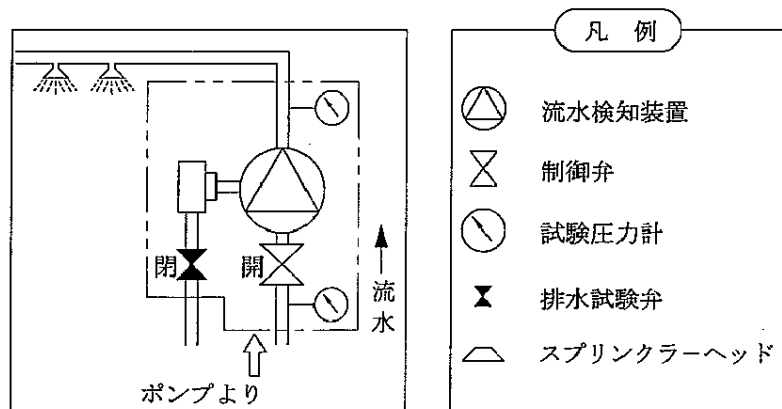
図6 流水検知
