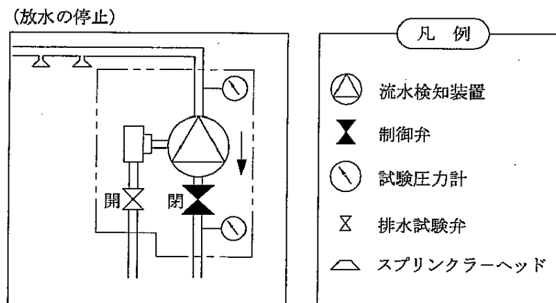
図12 二次側配管部の排水
