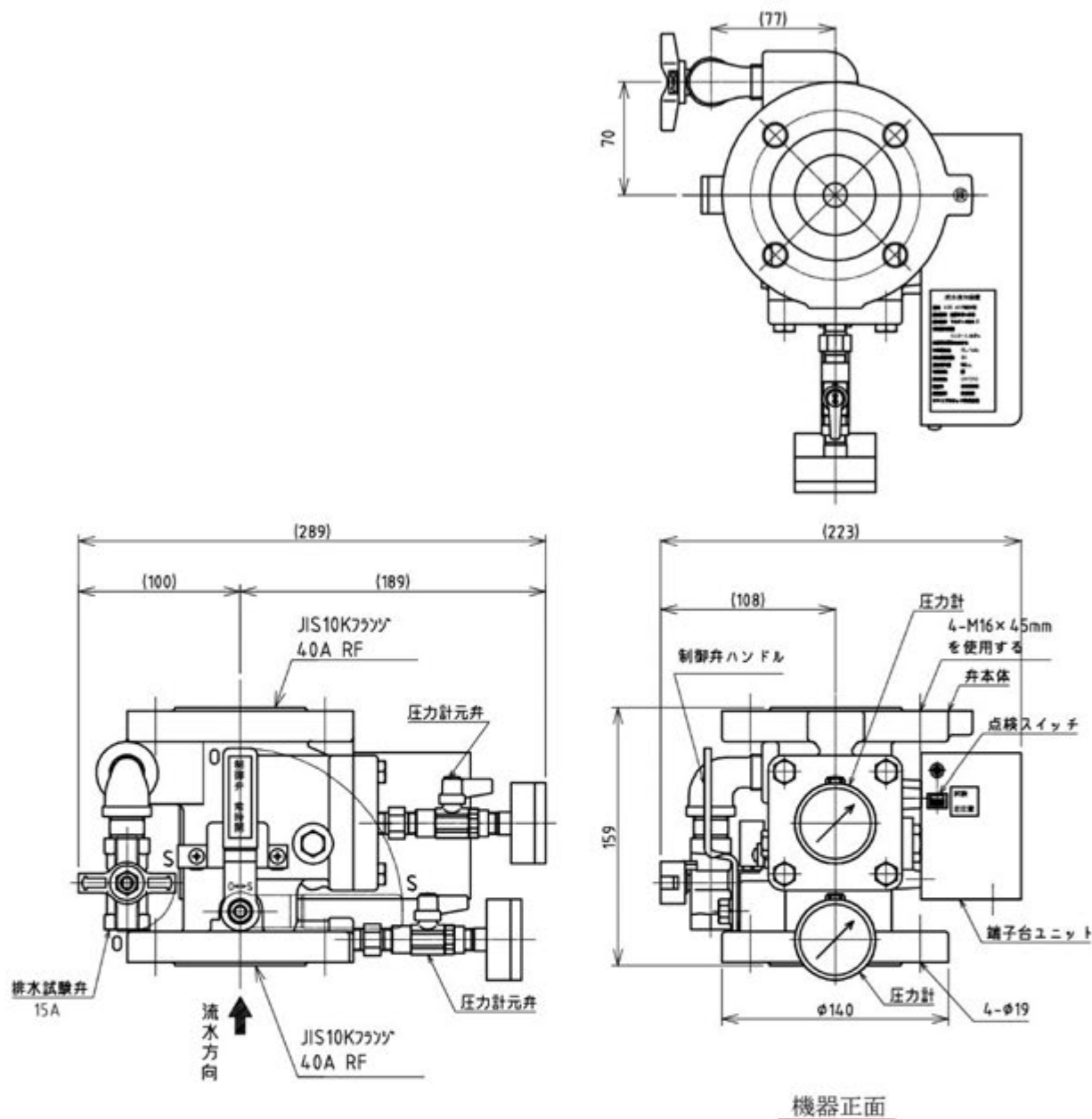
図 1 ユニット構成品の名称、外観寸法
