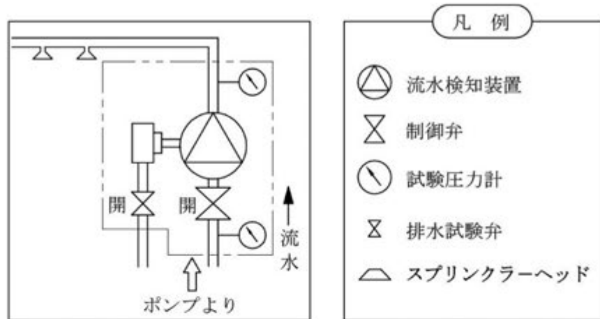
図 10 末端試験
