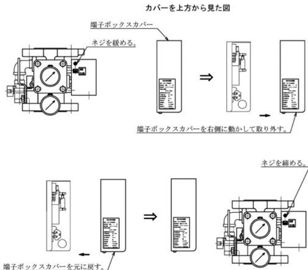
図5 端子ボックスのカバー脱着方法
