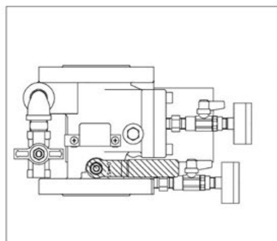
放水停止時
