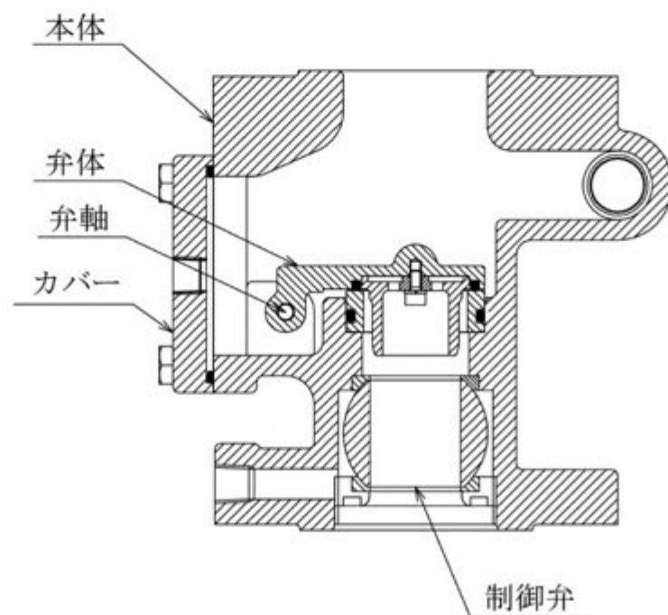
図 3 弁本体
