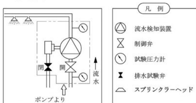
図6 流水検知
