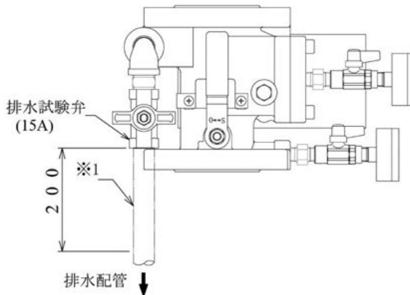
図 15 排水用配管の接続
