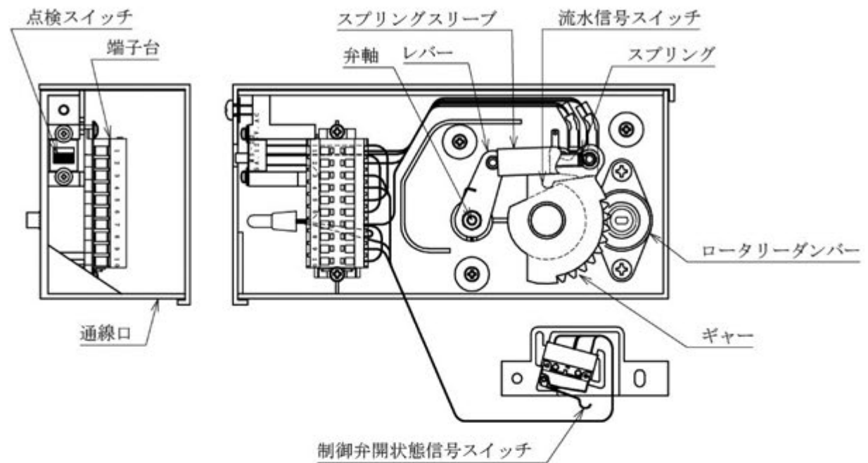
図 2 端子台ユニット
