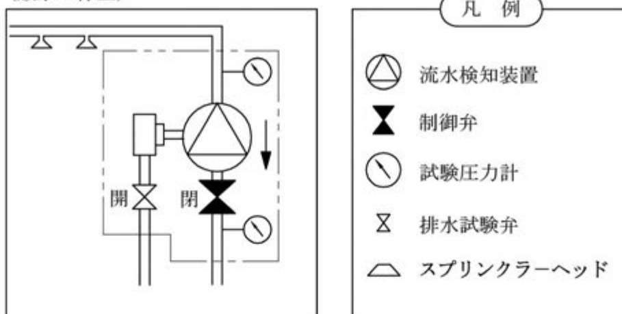
図 12 二次側配管部の排水
