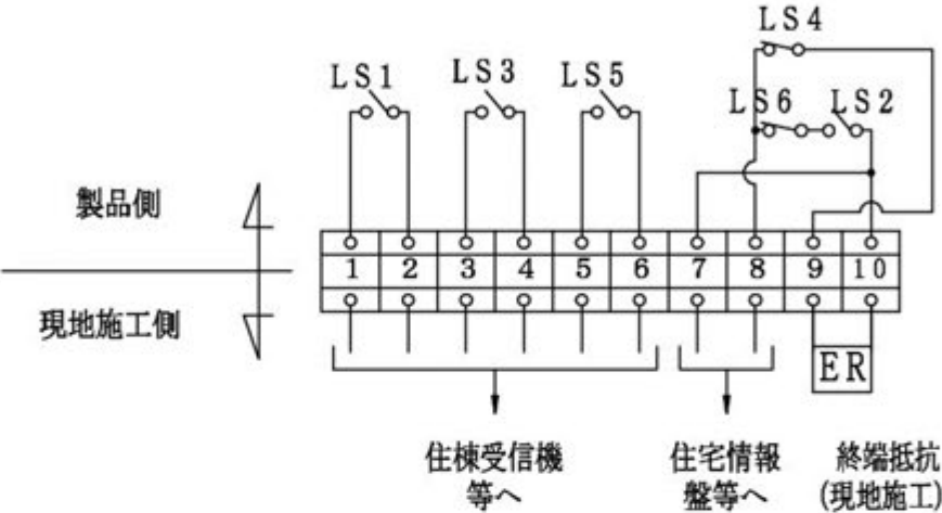
図 14 端子台ユニット結線図
