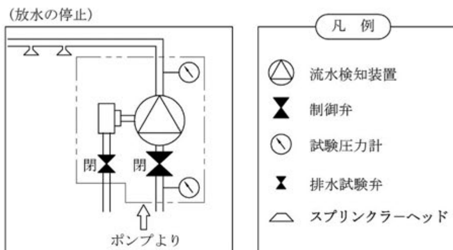
図8 放水の停止
