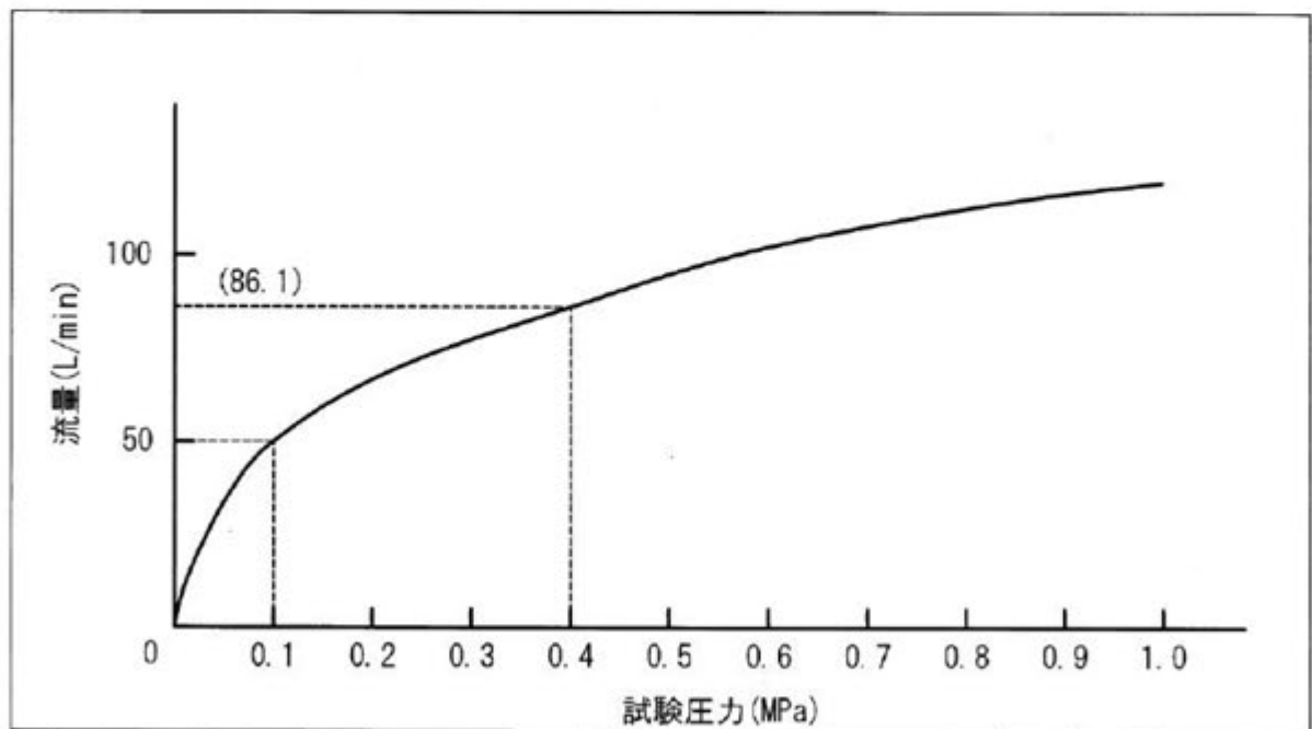
図 11 P-Q 線図
