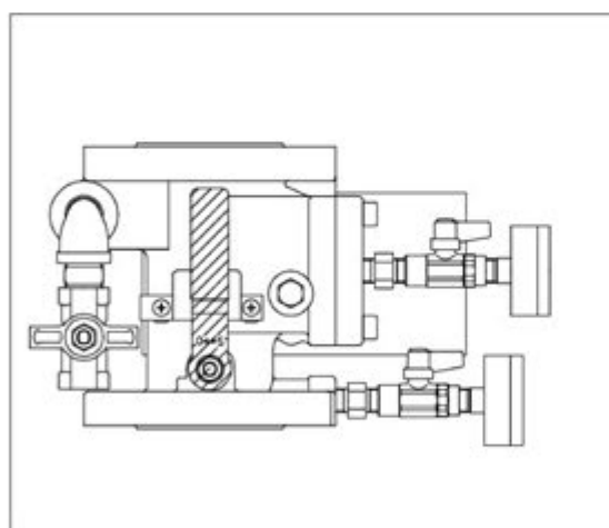
放水時
