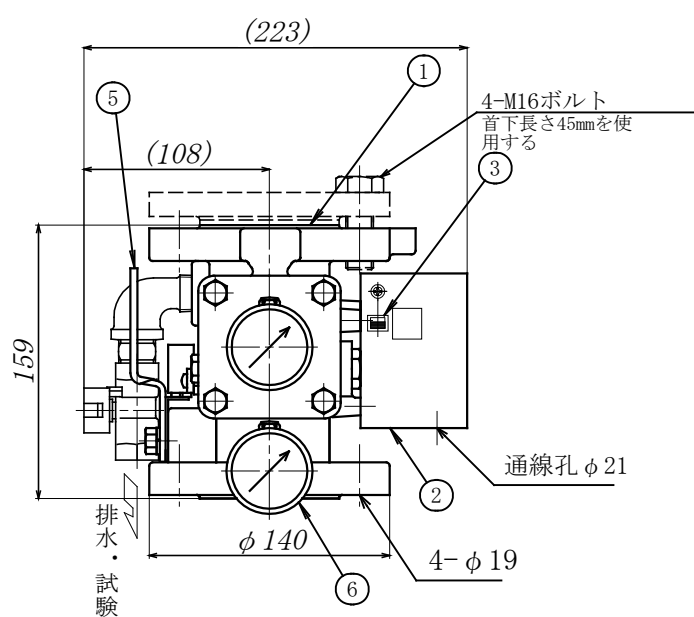
機器正面
