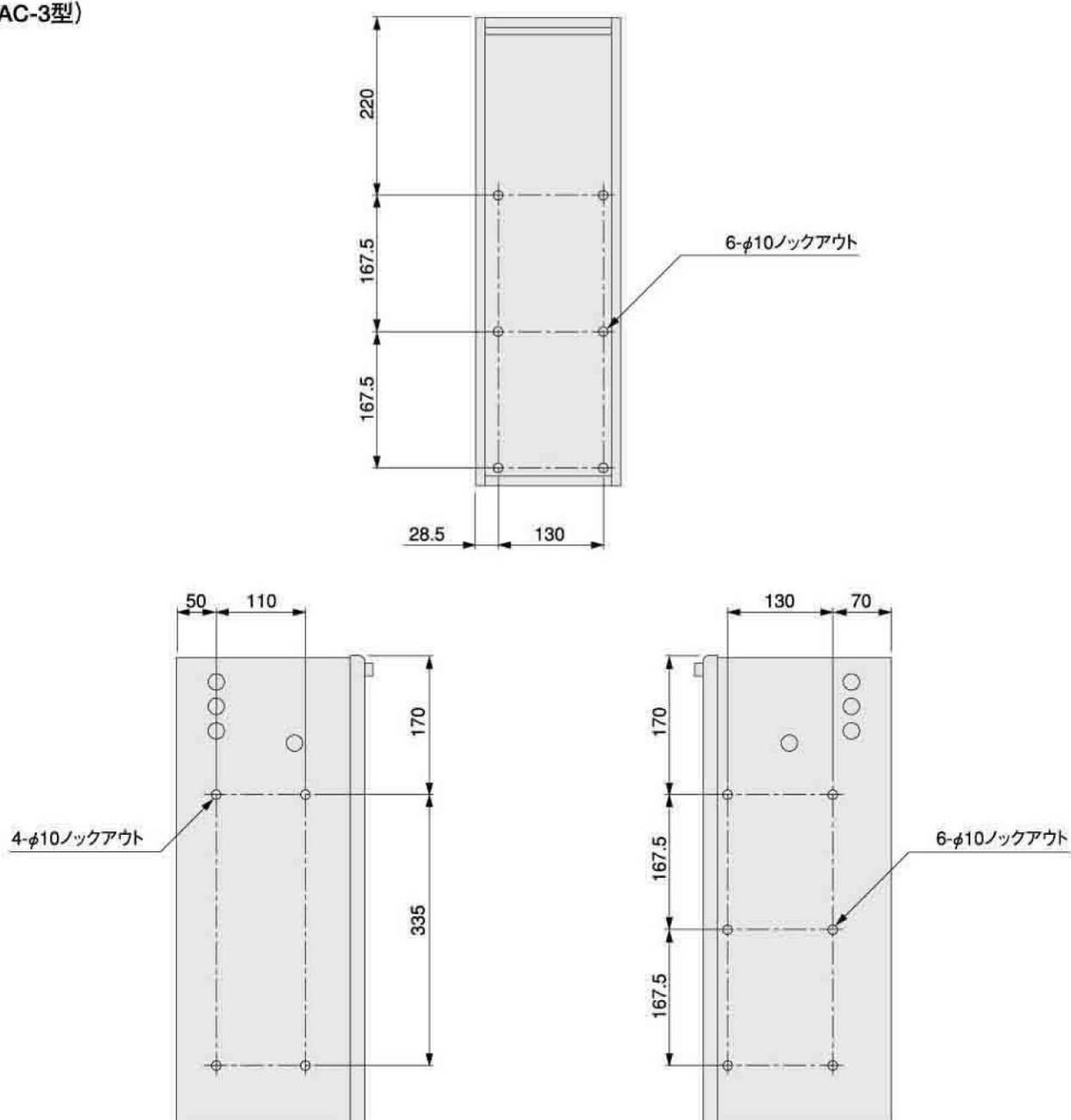
キャビネット取付穴寸法 (YAC-3型)
