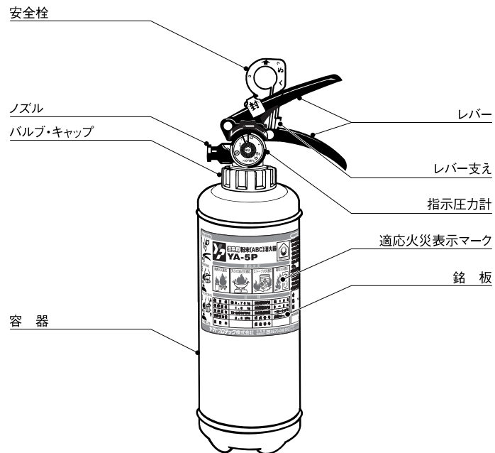
■住宅用粉末（ABC）蓄圧式消火器 YA-5P
