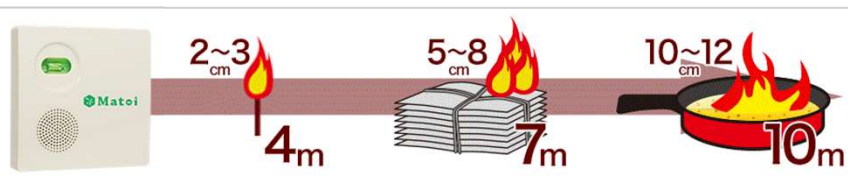
UVS-05BS-01・UVS-C 検知エリア図
