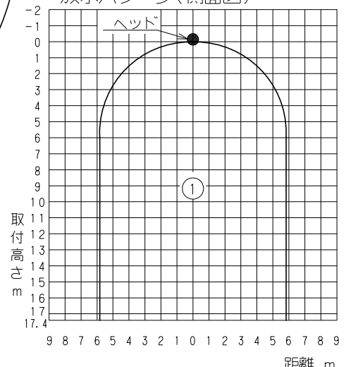
有効放水範囲 ① 5≤H≤17.4
