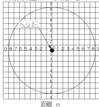
有効放水範囲 ① 5 \leq H \leq 17.4
