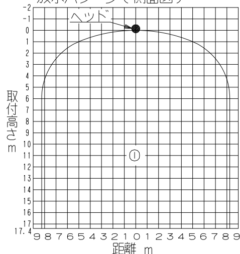
放水パターン (側面図)
