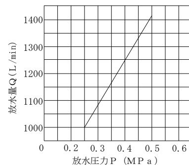
放水量特性 P-Q 曲線 Q=K\sqrt{10P}
