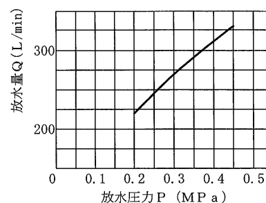
放水量特性 P-Q 曲線
