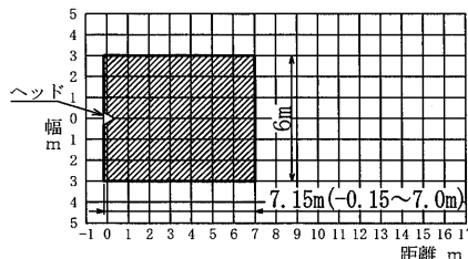
有効放水範囲
