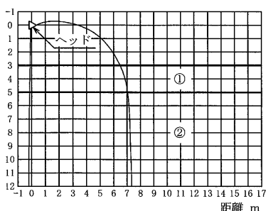
放水パターン (側面図)
