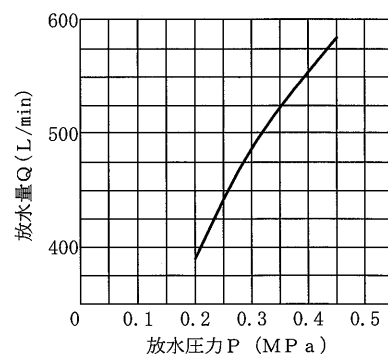
放水量特性 P-Q 曲線
