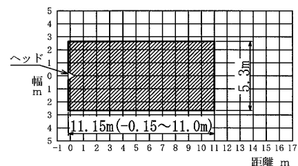
有効放水範囲 ② 5 \leq H \leq 12
