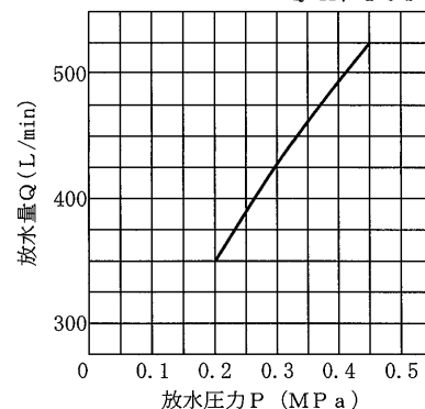
放水量特性 P-Q 曲線
