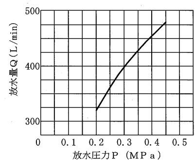
放水量特性 P-Q 曲線
