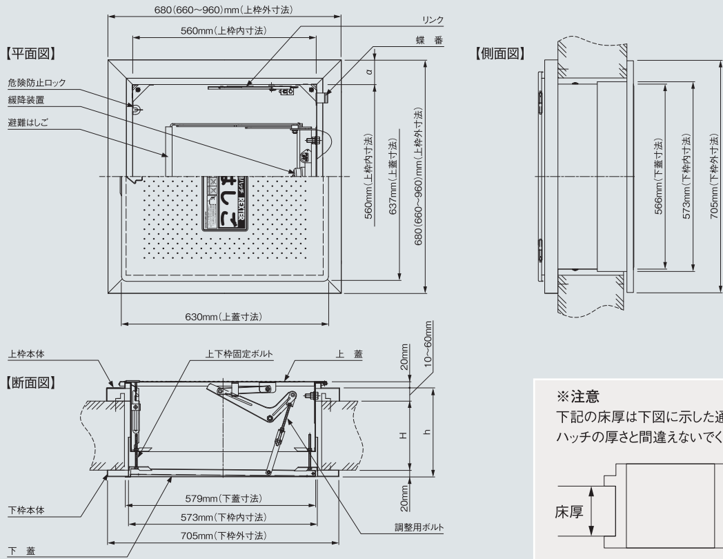
標準型(かさ高40mm) (単位:mm)
