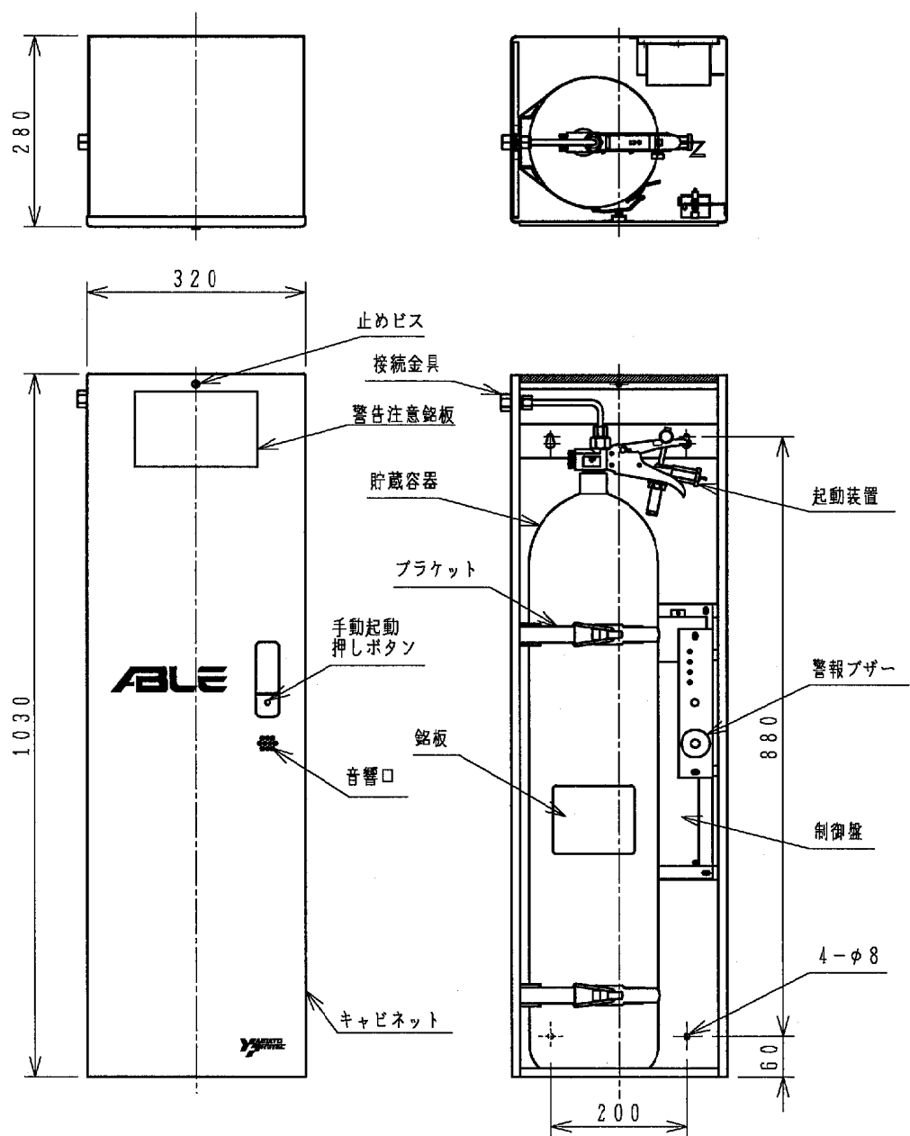
ACO-30B 外観図・内部配置図
