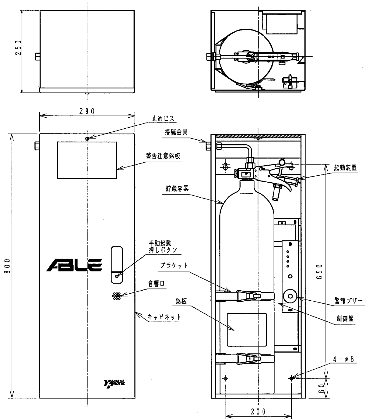
ACO-15B 外観図・内部配置図
