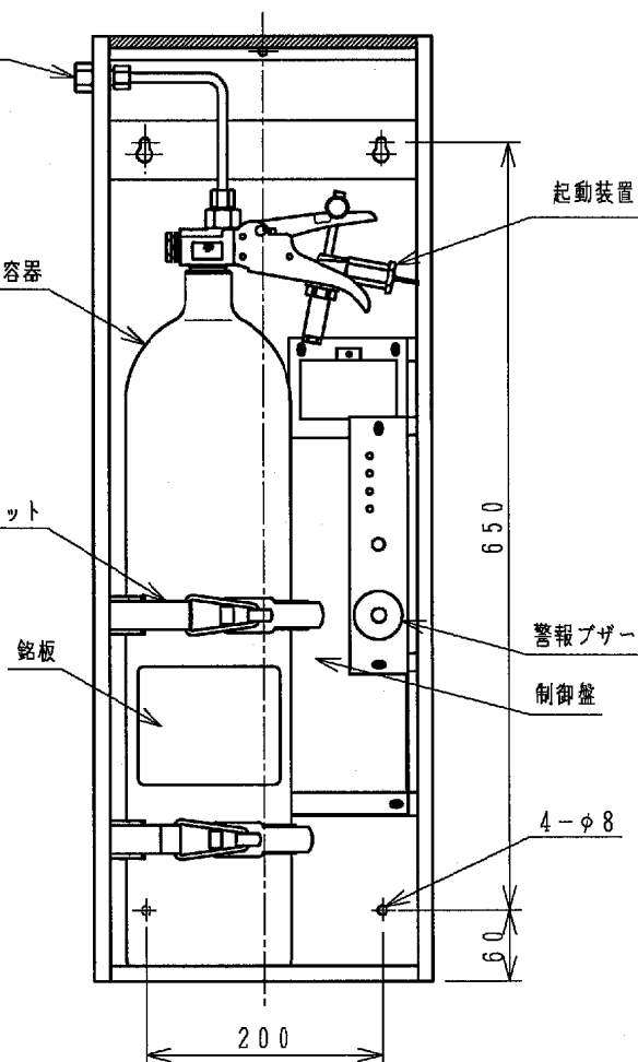
ACO-10B 外観図・内部配置図
