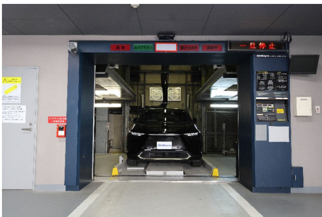
機械式駐車設備 入口外観
