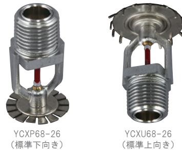
閉鎖型泡水溶液ヘッド
