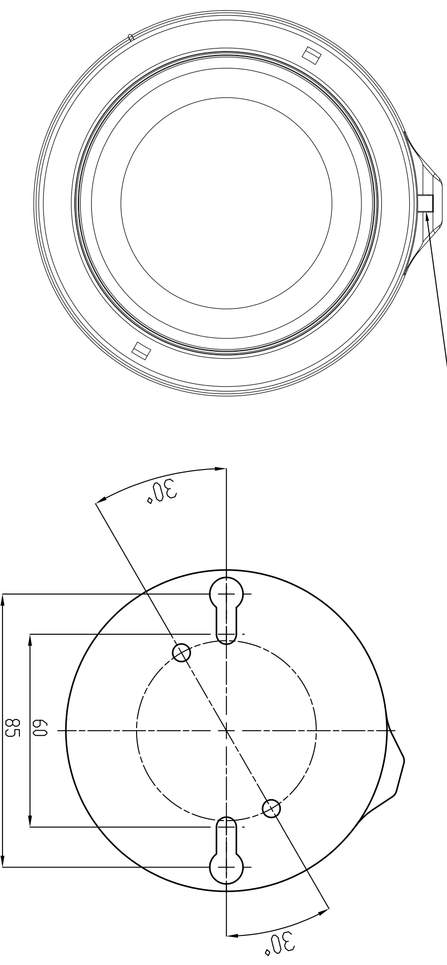
取付穴図 (天井側)
