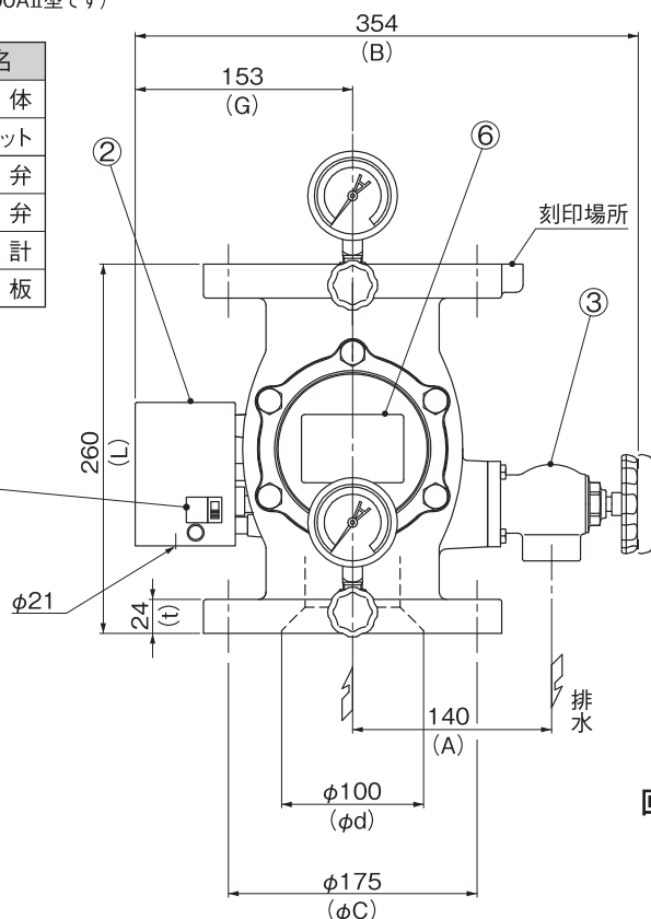
構造図 (図はYAVS-100AⅡ型です)
