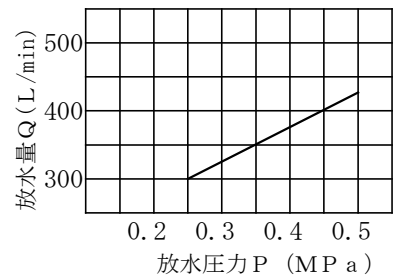
放水量特性 P-Q 曲線
