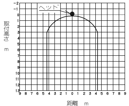
放水パターン (側面側)
