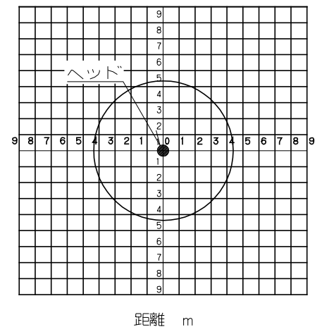
有効放水範囲 6 ≤ H ≤ 13
