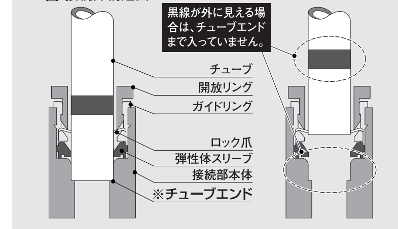
※A図:接続部構造図
