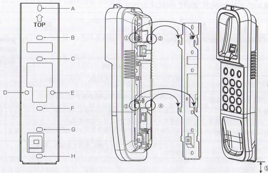
【壁掛け金具穴位置寸法】
