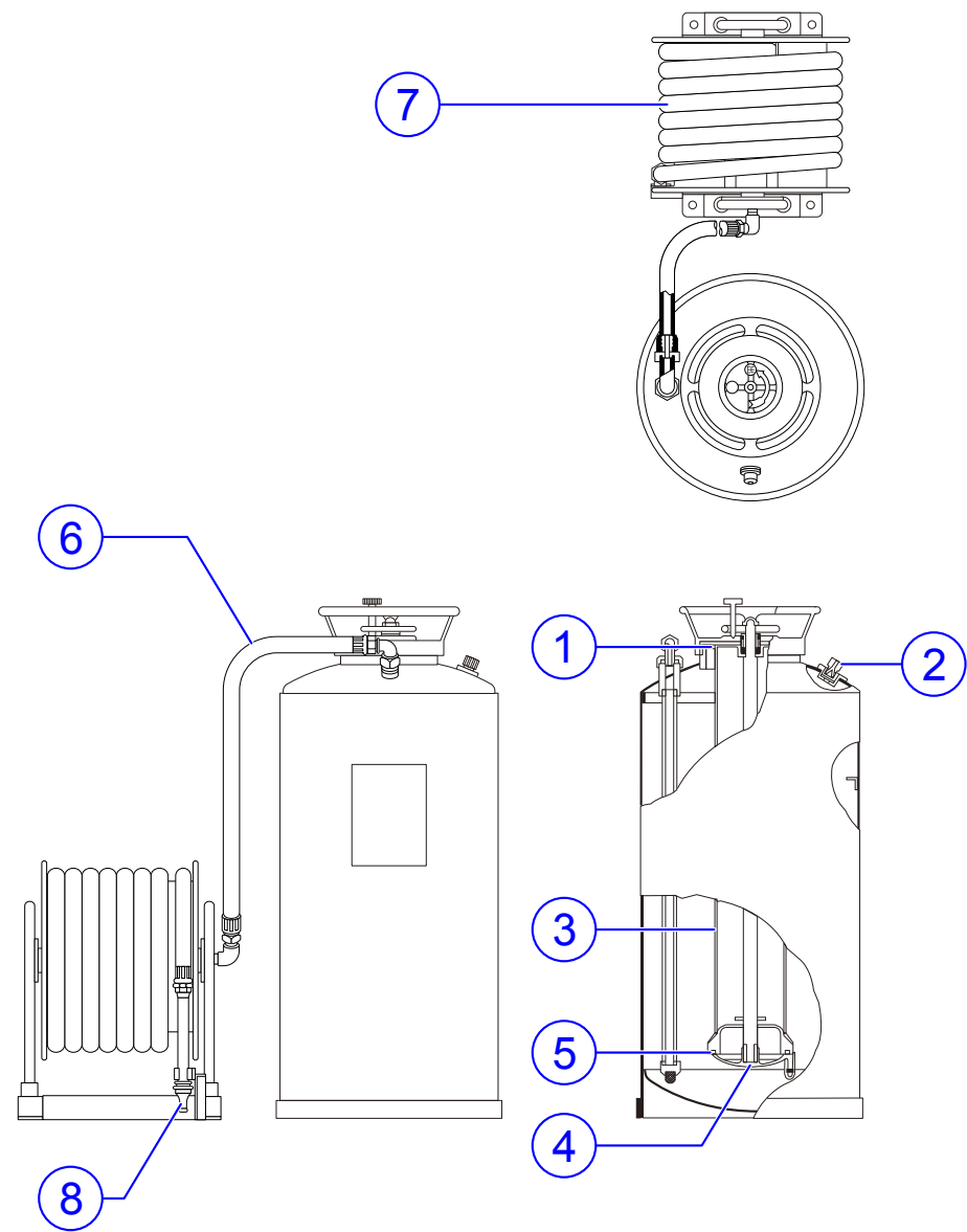
SF-150H 部品表
