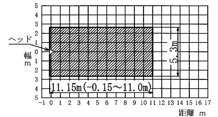
有効放水範囲 ② 5 \leq H \leq 12
