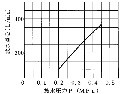
放水量特性 P-Q 曲線
