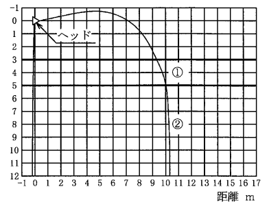
有効放水範囲 ① 3 \leq H < 5
