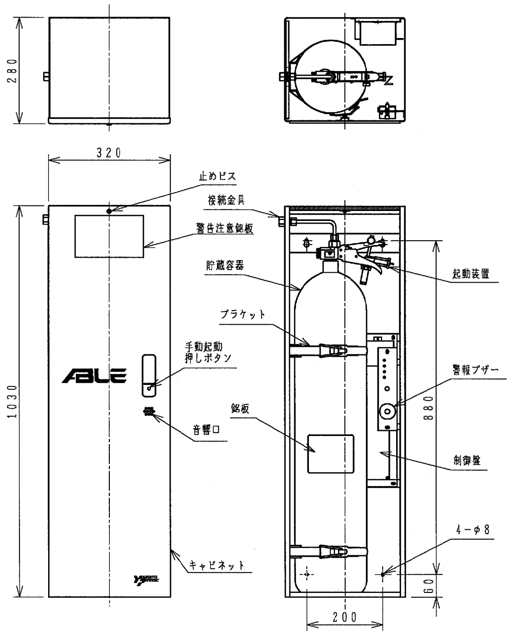
ACO-30B 外観図・内部配置図
