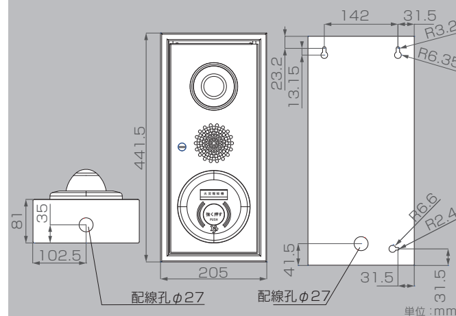
機器図
