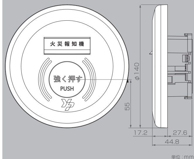
機器図
