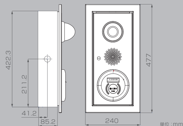
機器図
